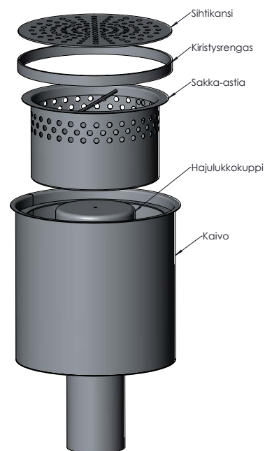
Kuvassa pönttökaivo 9083/1
